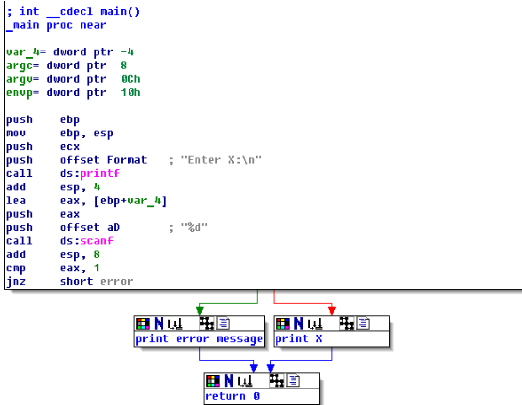
Fig. 1.19: IDA en mode graphe avec 3 nœuds reliés
