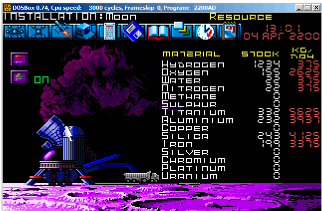
Fig. 9.18: Vérifions la valeur pour l'hydrogène
