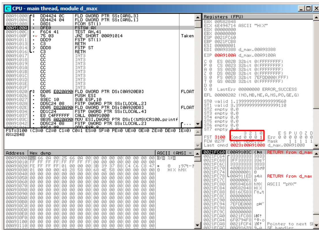
Рис. 1.78: OllyDbg: FCOM исполнялась
