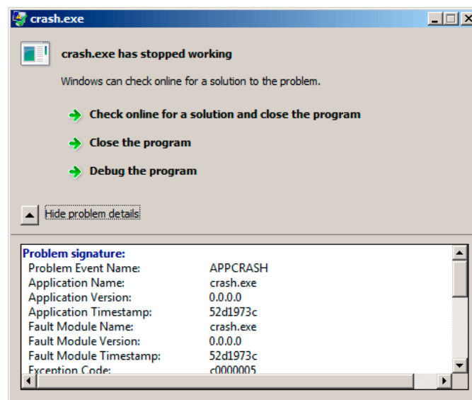
Рис. 6.4: Windows 7
