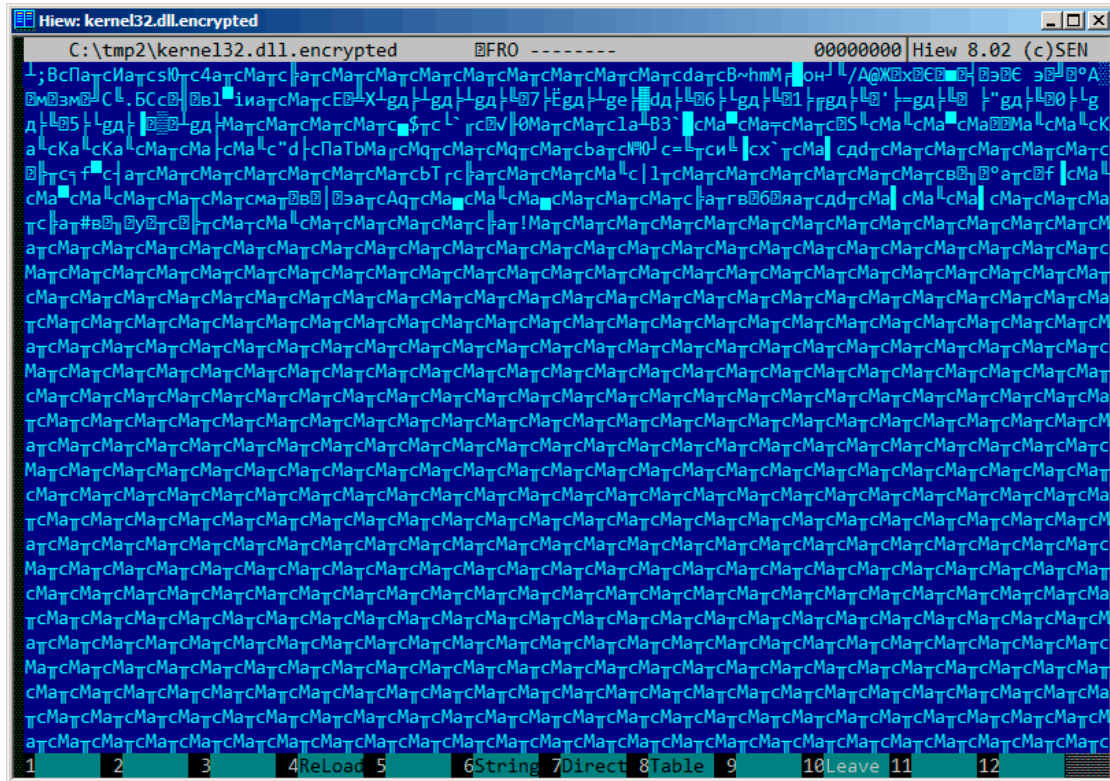
Рис. 9.5: «Зашифрованный» файл
