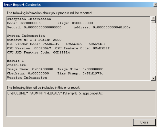
Рис. 6.3: Windows XP
