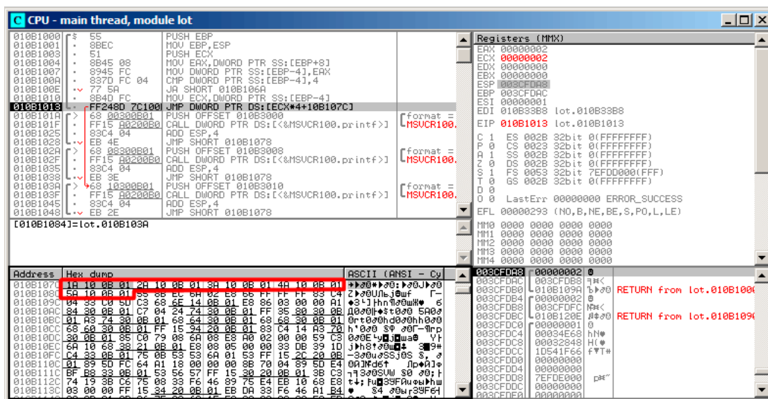
Рис. 1.52: OllyDbg: вычисляем адрес для перехода используя jumptable
