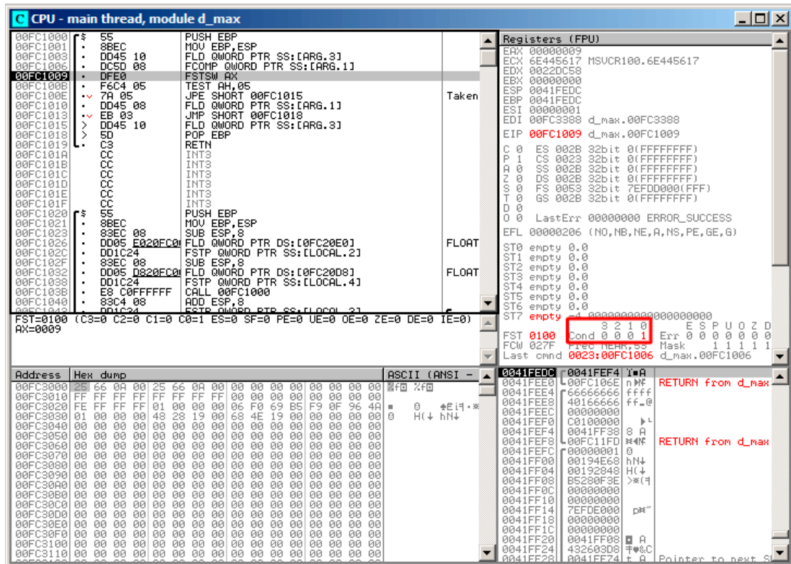
Рис. 1.73: OlyDbg: FCOMP исполнилась
