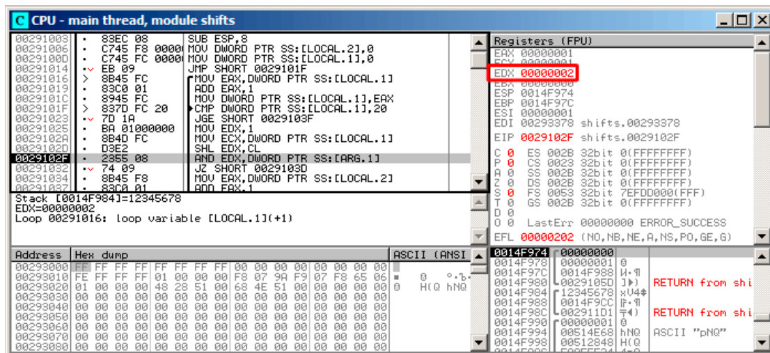
Рис. 1.99: OllDbg: i = 1 , EDX = 1 \ll 1 = 2
